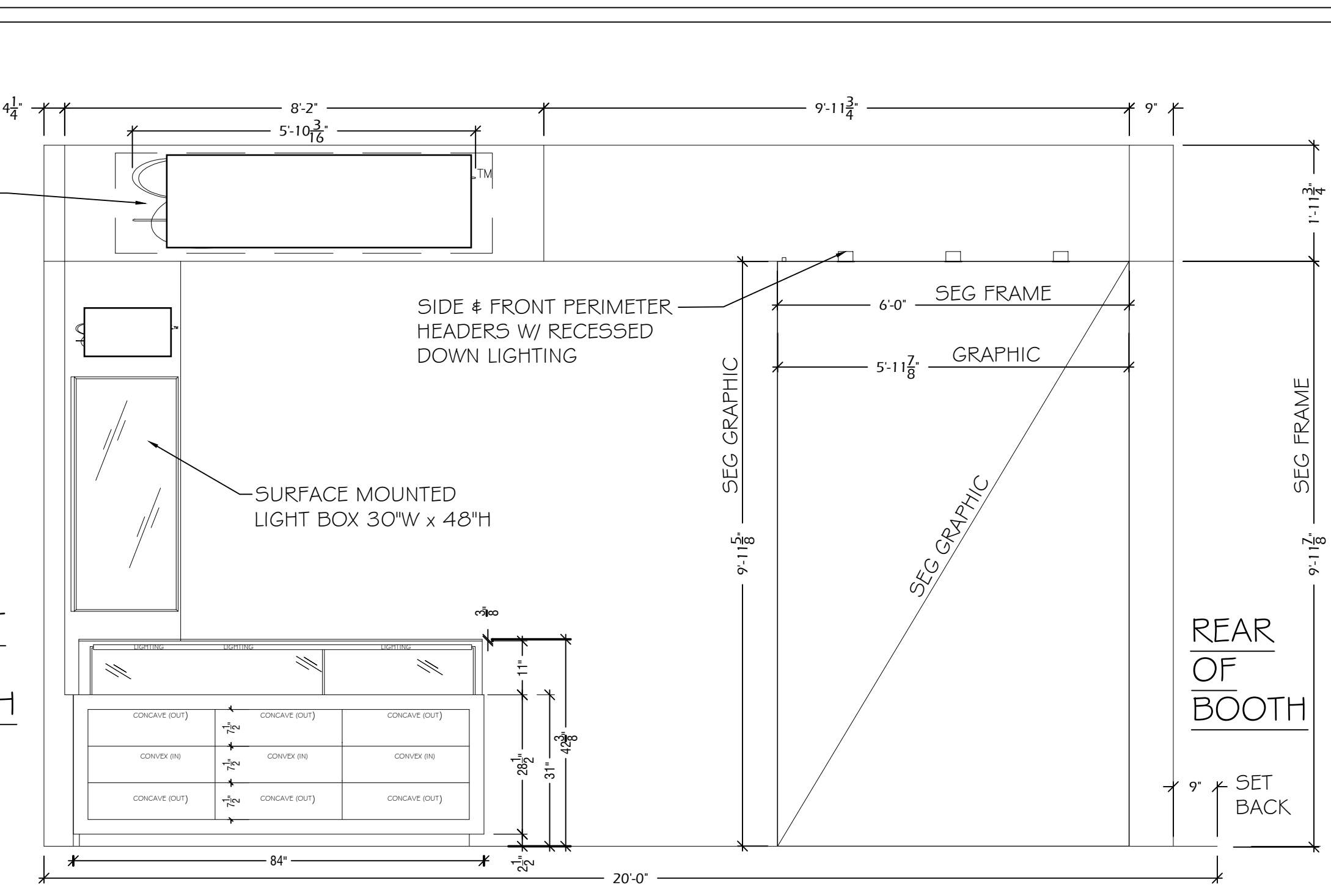
4 ELEVATION SCALE: 1/2"=1'-0"
