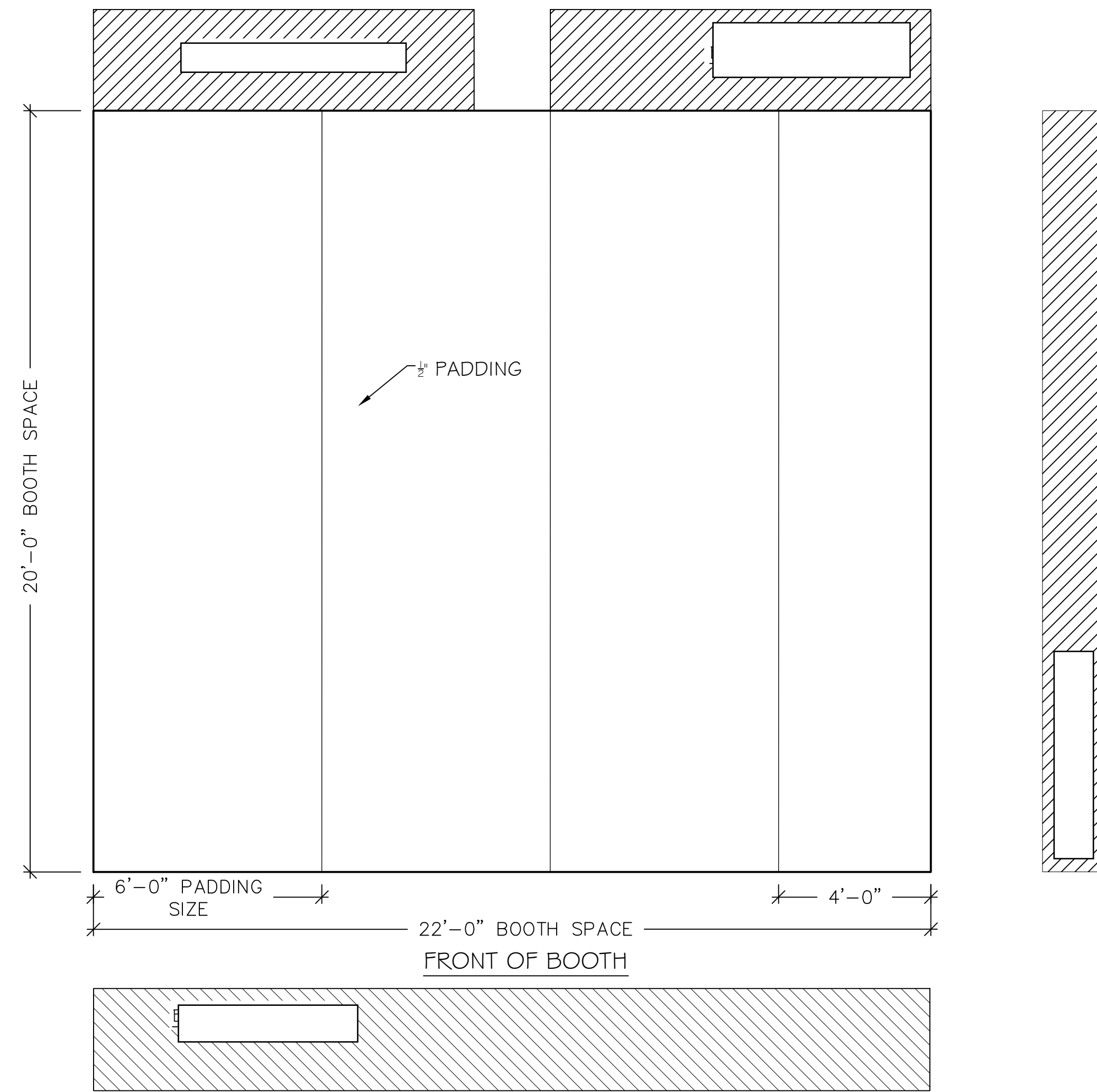
2 PADDING PLAN SCALE: 3/8"=1'-0"
